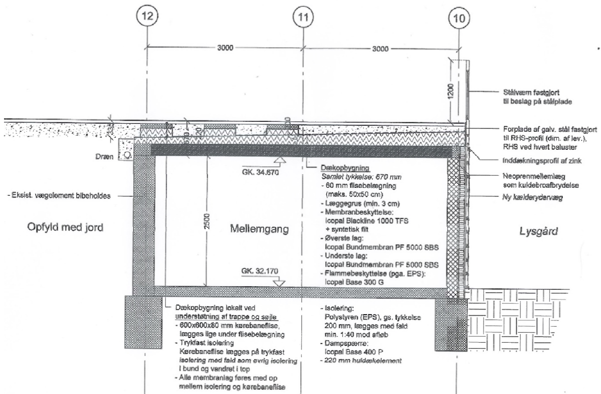
Figur 3.19: Snit i mellemgangen.
