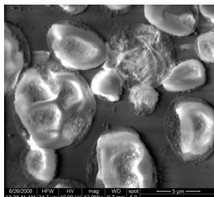
Prøve C: PCM stødt i morter og derefter i 0.1M NaOH i 2.5 time.
