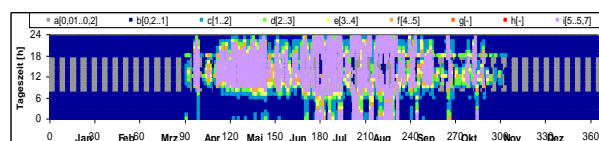
Figur 19. Luftsifte [h -1 ] over året for 'PCM' modellen.
