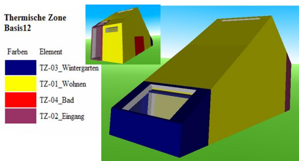
Figur 15. VRML præsentation som viser de termiske zoner i BSim modellen (fra 3D Thermal-View).
