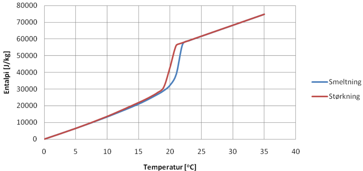
Figur 3. Enthalpi som funktion af temperaturen for PCM med smeltepunkt på 23 °C.
