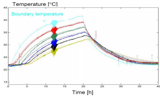
Figur 7. Test B. Knude 2 bruges som randbetingelse.
