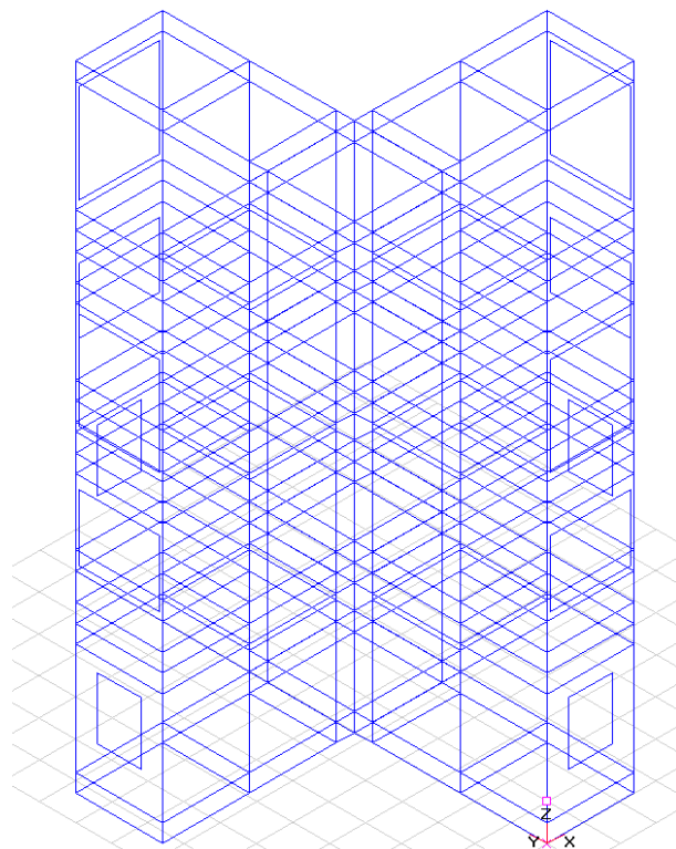
Figur 6. BSim model anvendt i analyse.
