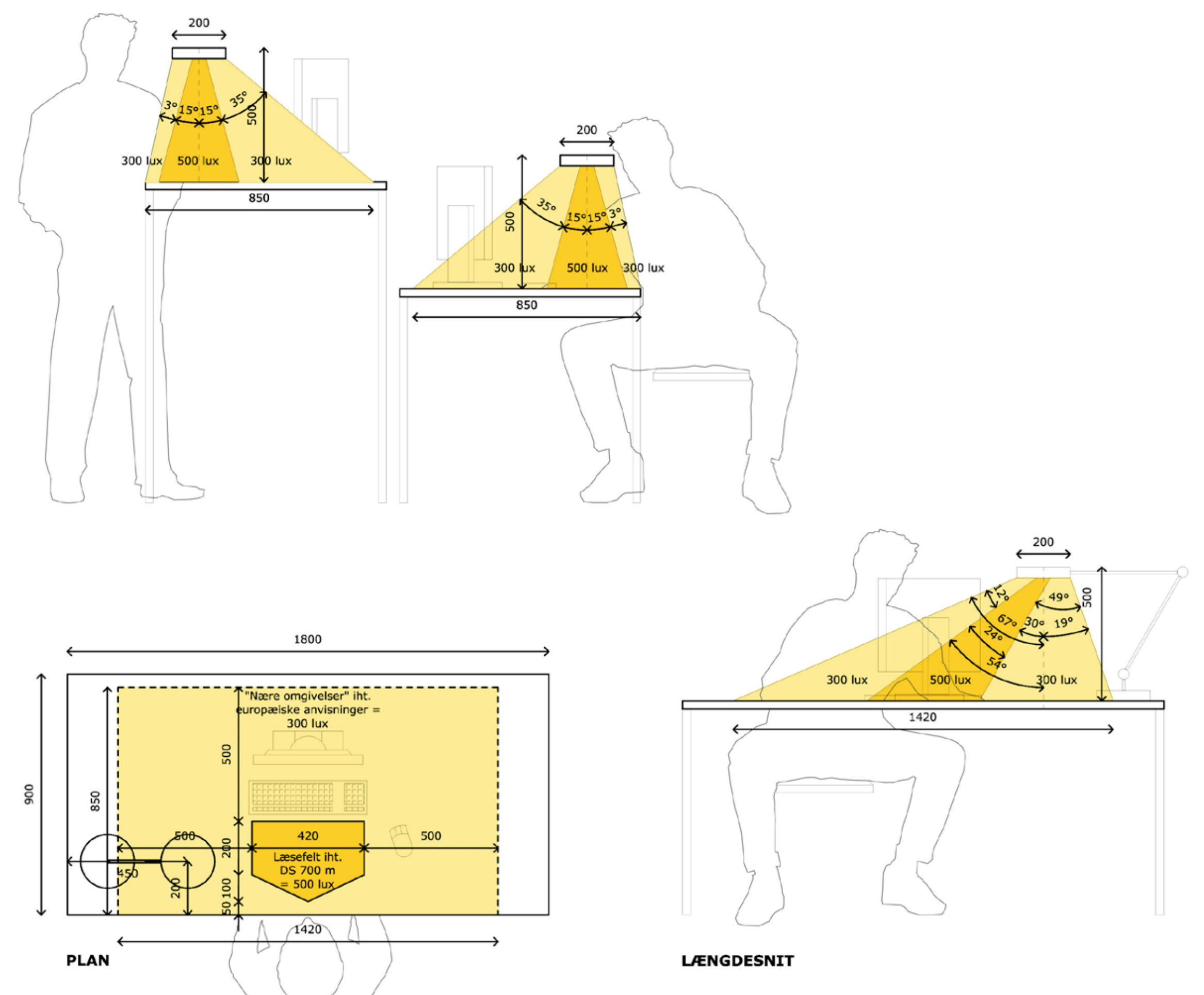
Belysningsareal 500 lux: Ifølge DS 700 Belysningsareal 300 lux: 500 mm omkring 500 lux areal Armaturstørrelse: Ø 200 mm Armaturhøjde: 500 mm Armatur placering: Midt udfør 500 lux felt
