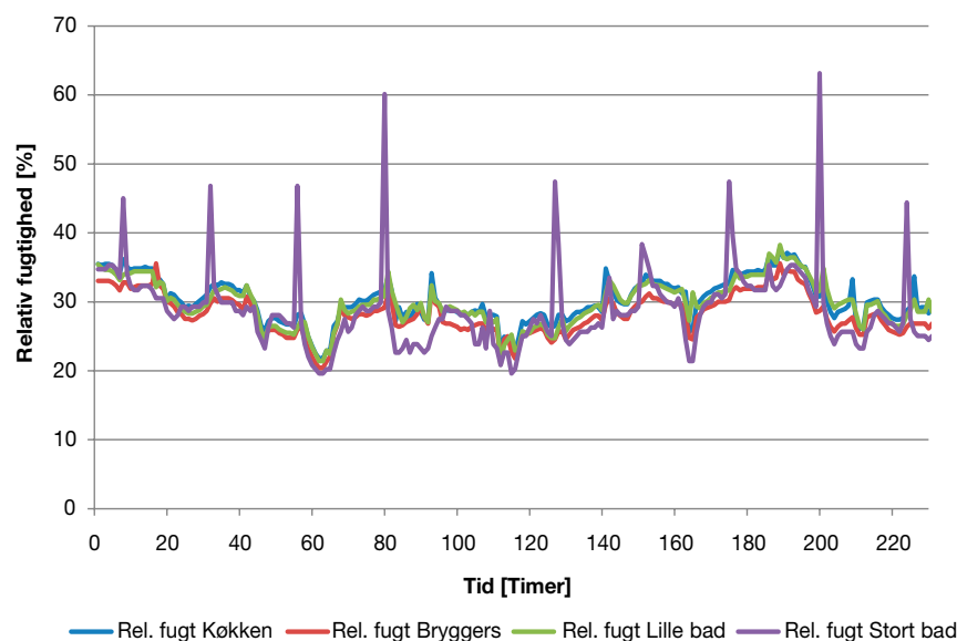
Figur 4. Den relative fugtighed i boligen når den simple regulering er i drift. Det ses, at fugten produceret om morgenen fjernes effektivt og at reguleringen ikke giver anledning til for høj relativ fugtighed i dagtimerne hvor ventilationsmængden er lav. De lave værdier skyldes, at målingerne er foretaget om vinteren.
