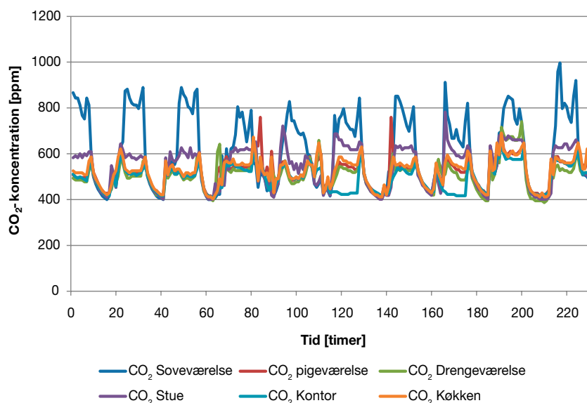
Figur 3. CO 2 -koncentrationen i boligen når den simple regulering er i drift. Sammenlignes med figur 1 ses, at reguleringen ikke giver anledning til dårligere luftkvalitet.
