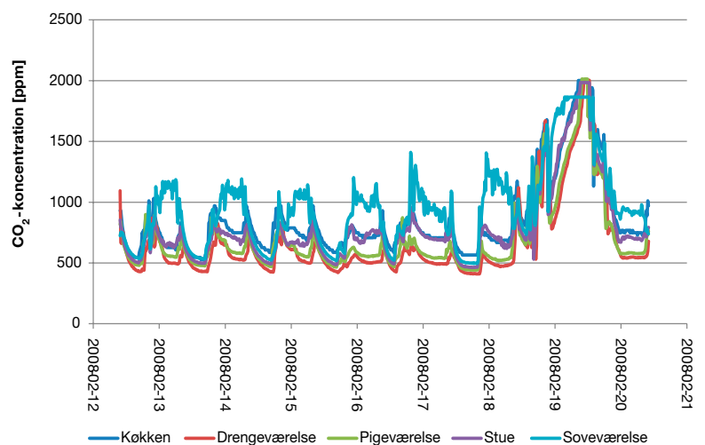
Figur 1. CO 2 -koncentrationen i boligen ved normal drift af ventilationsanlægget med konstant luftskifte. De sidste dage i måleperioden er ventilationsanlægget slukket. For at have acceptabel luftkvalitet anbefales CO 2 -koncentration under 1000 ppm.
