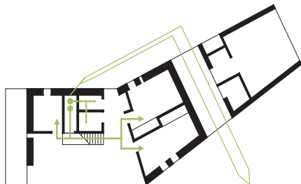
Fig. 2 Stueplan Ventilation Jordvarme
