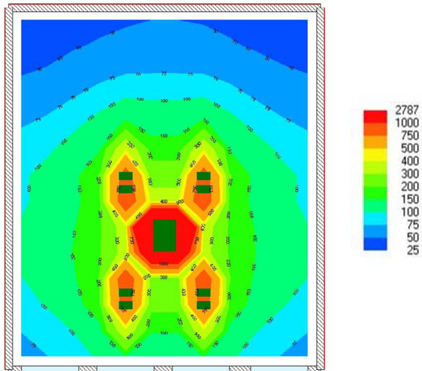
Figur 67: Belysningsstyrke (lux) på arbejdsplanet, hvor arbejdslamperne er suppleret med lys fra up-light stander
